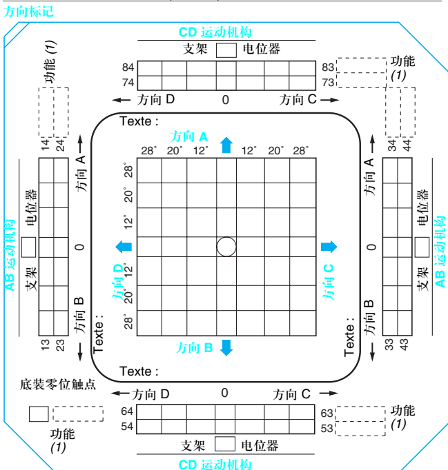
图 1：每运动机构 4 副触点 (顶视图)
