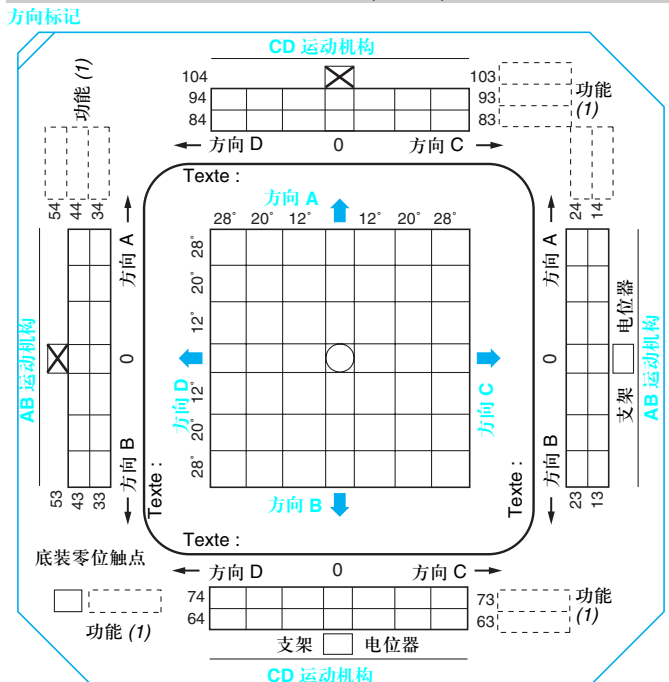
图 2：每运动机构 4 副触点 +1 副零位触点 (顶视图)
